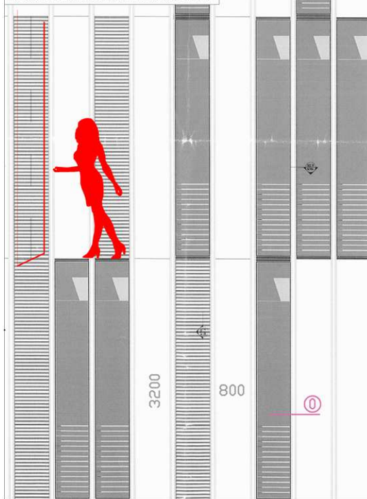
FACCIATA INFISSO MODELLO GIUDITTA
